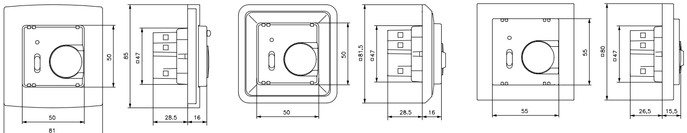
Regler 50 x 50 mit Alre-Rahmen Controller (50 x 50) with Alre type frame
