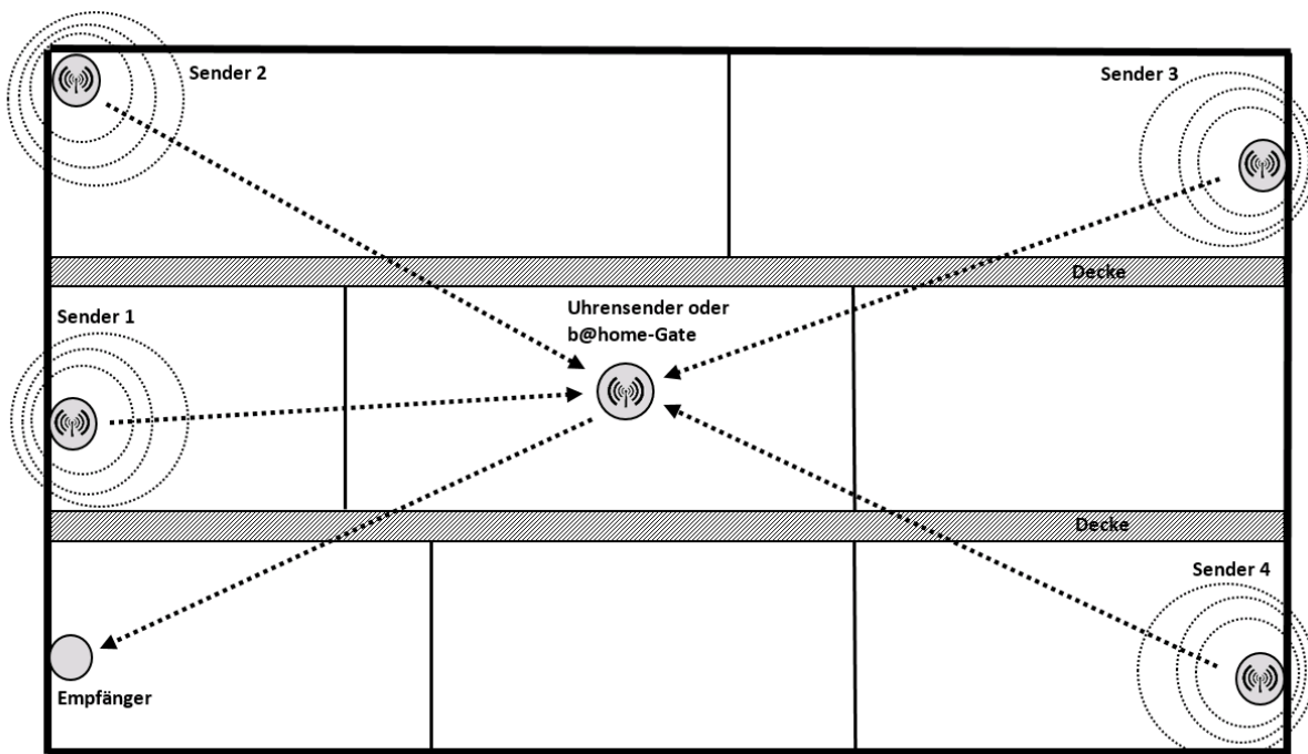
Hausquerschnitt mit zentral positioniertem b@home-Gate
