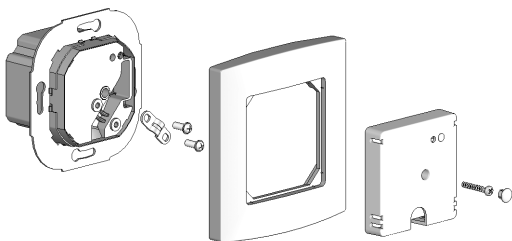
Regler 50 x 50 mit Rahmen
