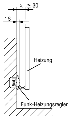
Montage hinter dem Heizkörper nur im unteren Kantenbereich.
