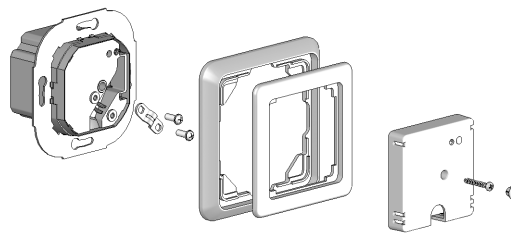
Regler 50 x 50 mit Beispiel-Rahmen und Zwischenrahmen
