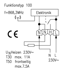
Anschluss-Zeichnung
