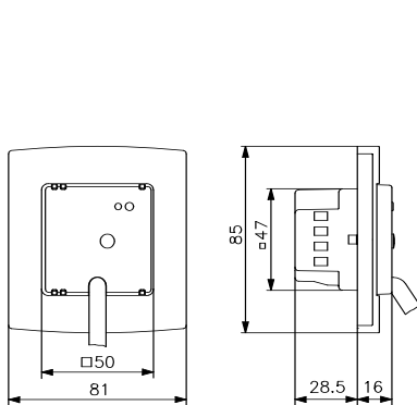
Regler 50 x 50 mit Rahmen
